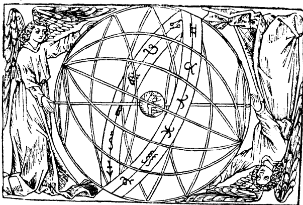
Рис. 4.15. Средновековни представи за вселената, тоест за небесния храм. Ангели въртят осите, колелата, зодиакалния кръг. От книгата на J. de Sacro Bosco „Opusculum Johannis de Sacrobusto spericum, cu figuris optimis ei novis textu in se, sive ambiguitate declarantibus“ – Leipzig, 1494 г. [1383]. Книгохранилището на Пулковската обсерватория (Санкт Петербург). Вж. също [543], с. 118, ил. 64.
