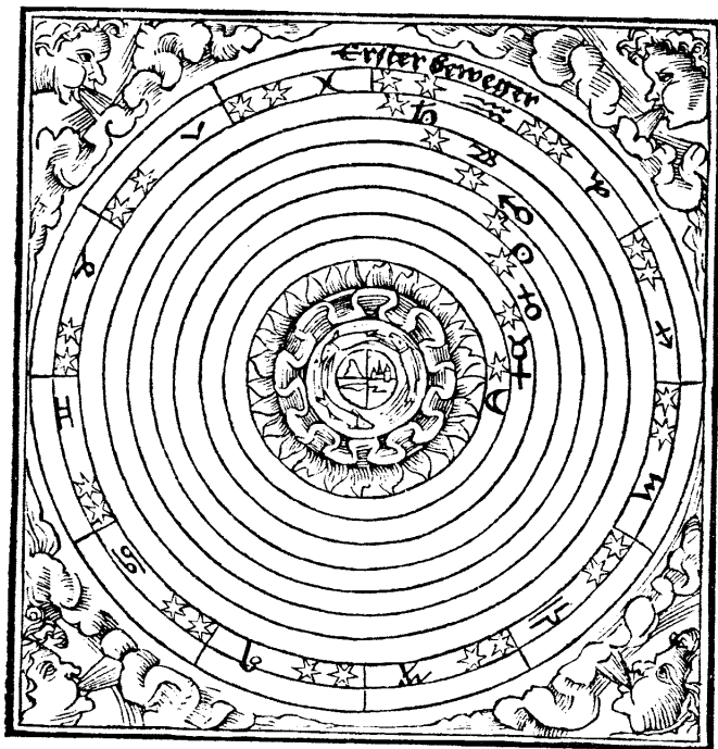
Рис. 4.5. Орбитите на планетите като колела в колелата. От средновековната книга на J. de Sacro Bosco (или Sacrobusto) „Sphera Materialis“, 1516 г. [1384]. Книгохранилището на Пулковската обсерватория (Санкт Петербург). Вж. също [543], с. 118, ил. 65.
