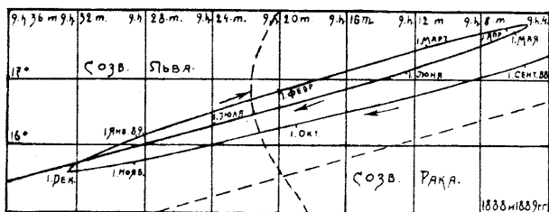
Рис. 3.20. Примкообразният път на Сатурн между съзвездията Рак и Лъв през 1888 и 1889 г. От [542], с. 12, ил. 4.
