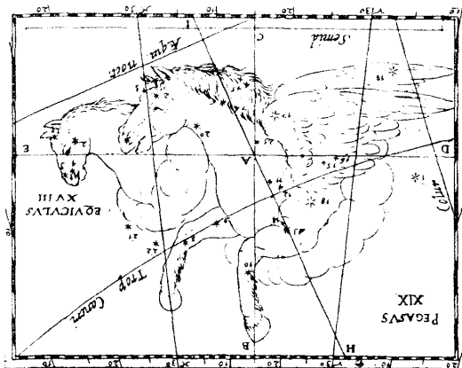
Рис. 3.19. Съзвездие Пегас в звездна карта в книгата „Grienberdera“ [1162]. Книгохранилището на Пулковската обсерватория (Санкт Петербург). Вж. също [542], с.
